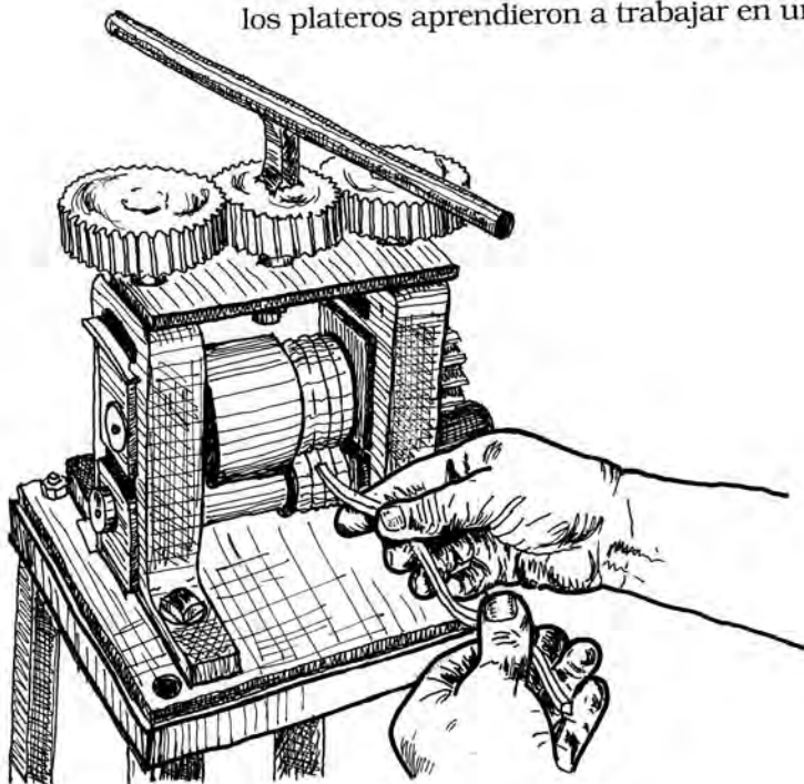
Laminador de alambre
